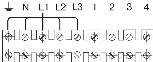
Рис. 5. Схема подключения HT 915
